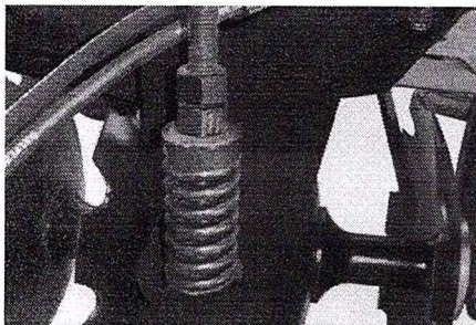
Mola estabilizadora. Stabilization spring. Resorte estabilizador.
